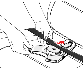
Шаг 2: Сдвиньте автомобильное крепление под ремнем в зацеп для ремня.
